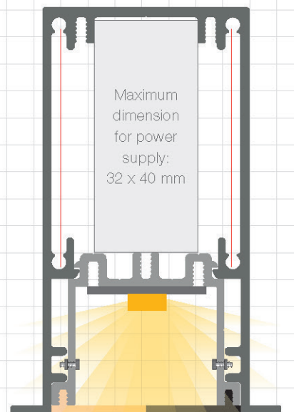
Moscu Magnum Slim easyON IP65 49,7 x 75 mm
