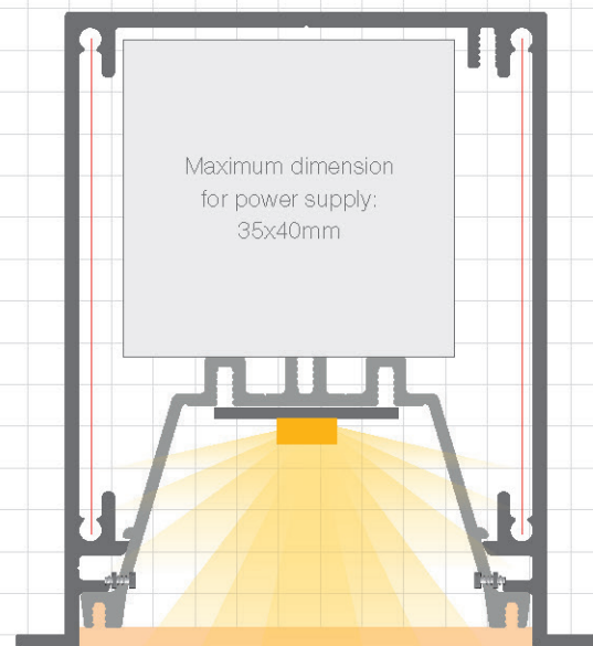
Moscu Magnum easyON IP65 72 x 76 mm
