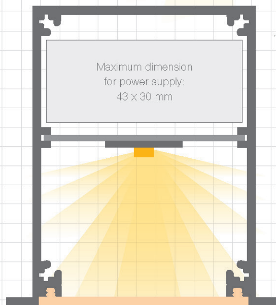
Moscu easyON IP65 72 x 78 mm
