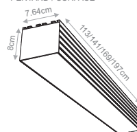
TETRA PLUS EM TRIMLESS PENTAND / SURFACE
