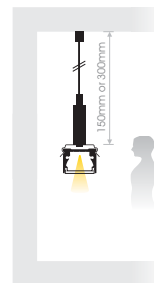
PENDANT installation
