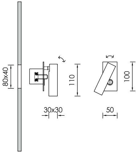
FERUS 60 H.P.LED
