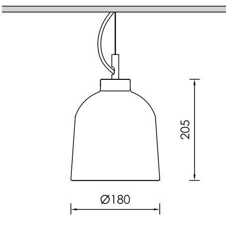
FUMO SP 4
