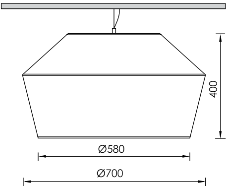
VERNO 60 LR
