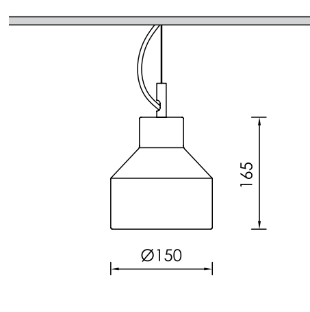
FUMO SP 6
