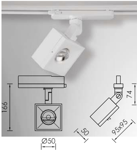
VELOX 5 Q
