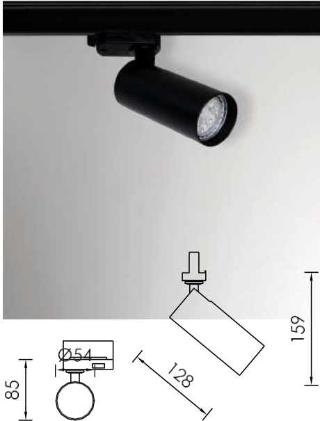
POTIS S
